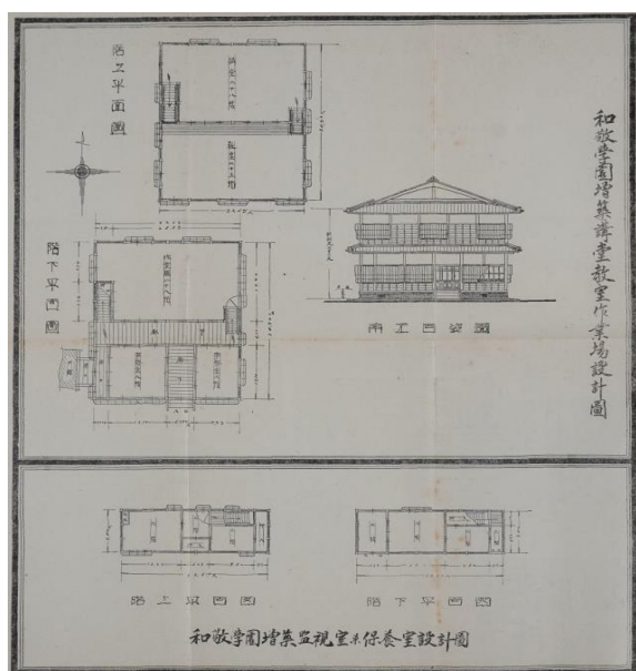
写真6 和敬学園新園舎設計図(『衆善』昭和8年6月号)
